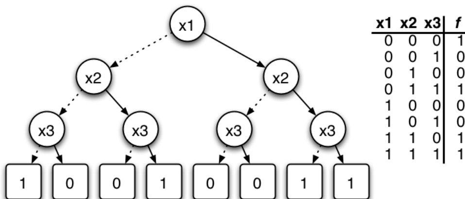
شکل ۱: درخت تصمیم دودویی و جدول ارزش برای تابع f: f(x_1, x_2, x_3) = (\neg x_1 \wedge \neg x_2 \wedge \neg x_3) \vee (x_1 \wedge x_2) \vee (x_2 \wedge x_3)
